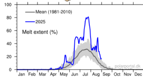
Melting
