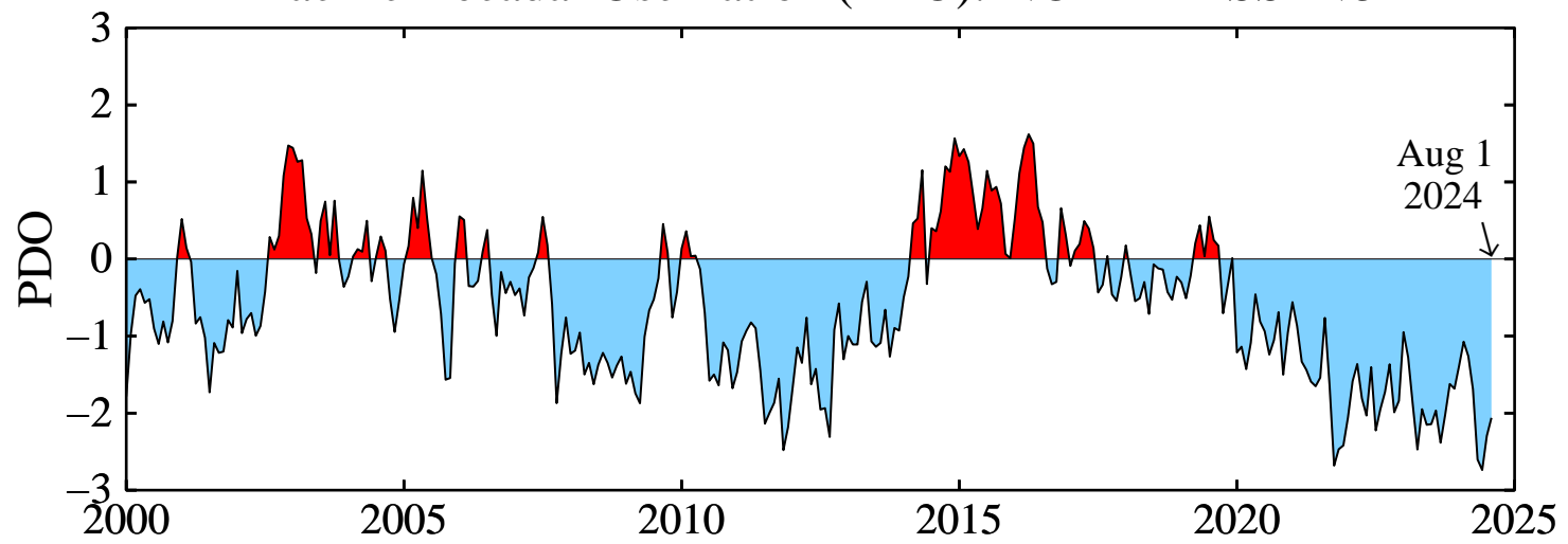
Pacific Decadal Oscillation (PDO): NOAA ERSST v5
